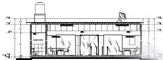
CORTE LONGITUDINAL 01
