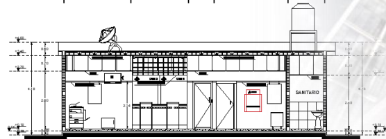
CORTE LONGITUDINAL 02
